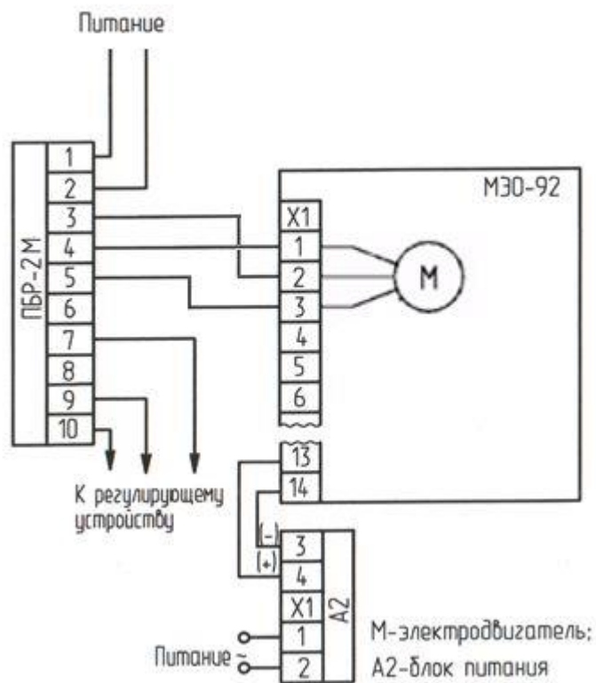
Рисунок Д.3 – Схема бесконтактного управления механизмом МЭО-92
