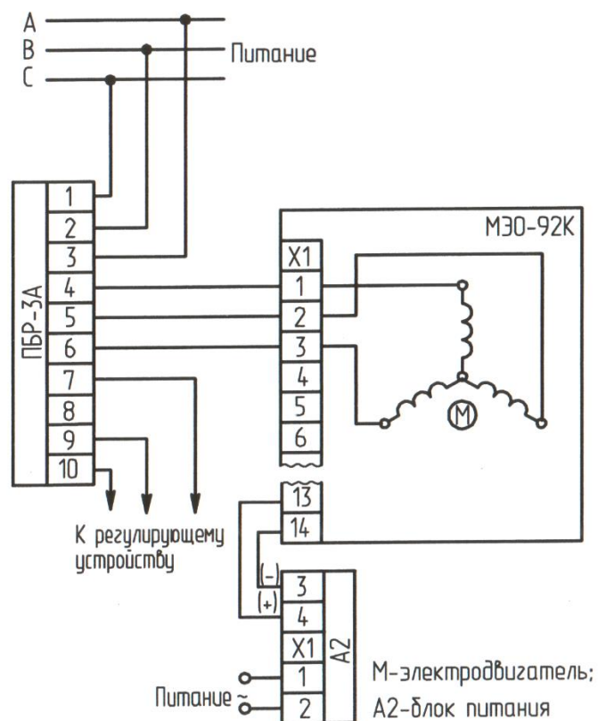
Рисунок Д.2 – Схема бесконтактного управления механизмом МЭО-92К
