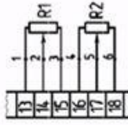
Рисунок Г.4 – механизмы с БСПИ-10 Остальное – см. рисунки Г.1
