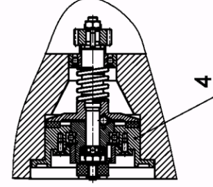
Рисунок Б.1 – Механизмы МЭО-1600 / МЭО-2500
